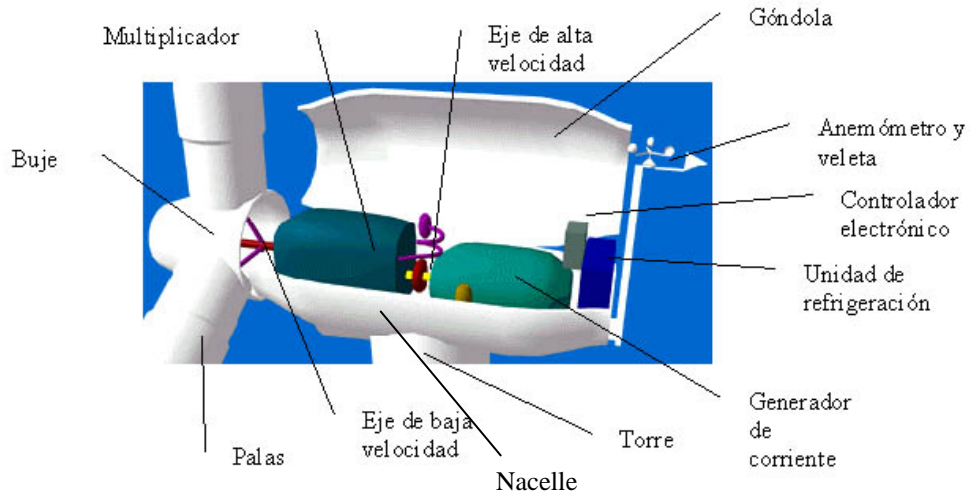
FIGURA 1 COMPONENTES AEROGENERADOR
